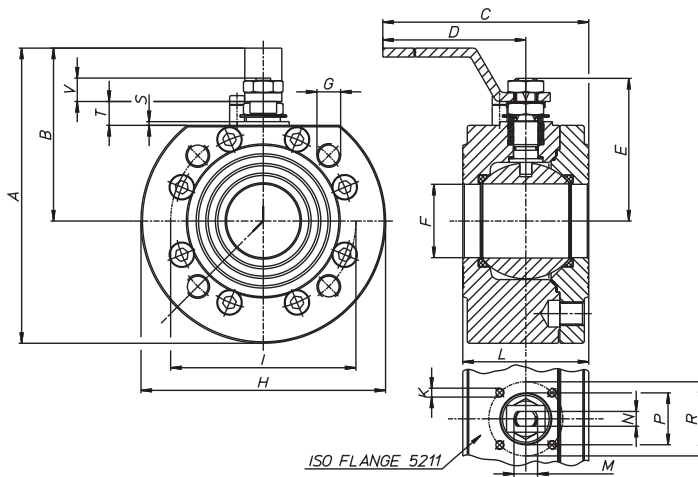
ISO FLANGE 5211
